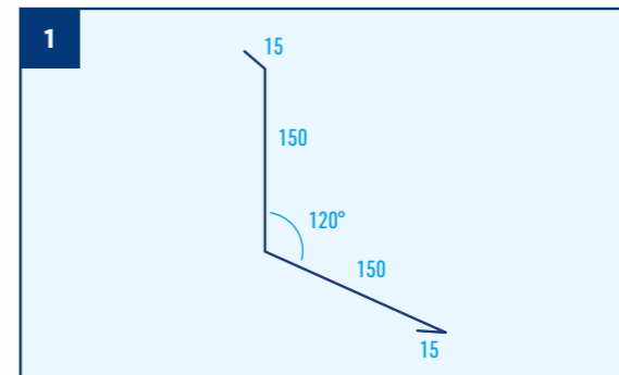
Lemování zdiva, r.š. 330 mm
