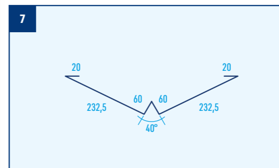
Lišta úžlabí se stojatou drážkou, r.š. 625 mm
