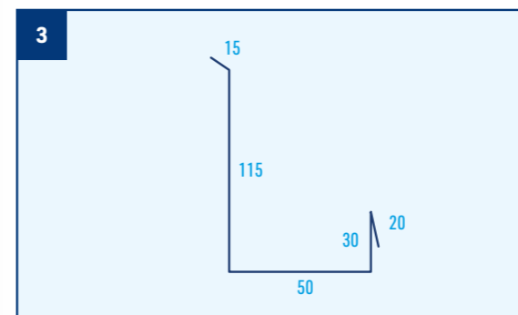
Lišta boční (plochá), r.š. 230 mm
