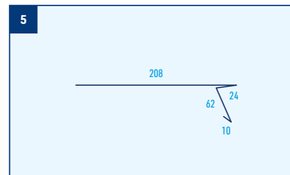
Lišta okapní, r.š. 304 mm
